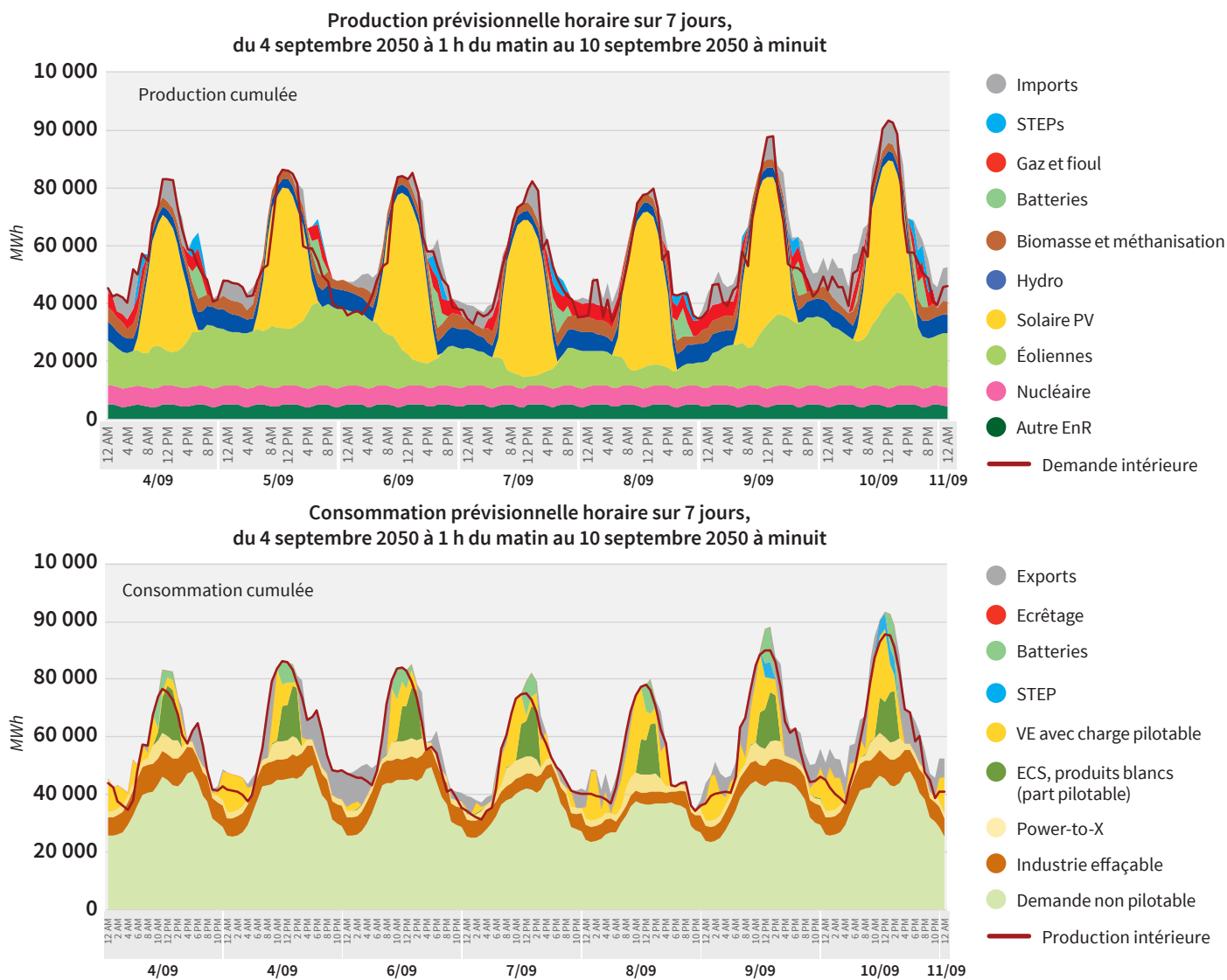
FIGURE 7 : EXEMPLE DE RÉSULTAT DU MODÈLE SUR UNE SEMAINE D'HIVER 2050 (EN HAUT, L'APPEL DES DIFFÉRENTS MOYENS DE PRODUCTION ; EN BAS, LA DÉCOMPOSITION DE LA DEMANDE) (21)
