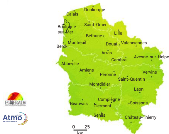
Concentrations en particules PM10 Moyennes annuelles de fond *
