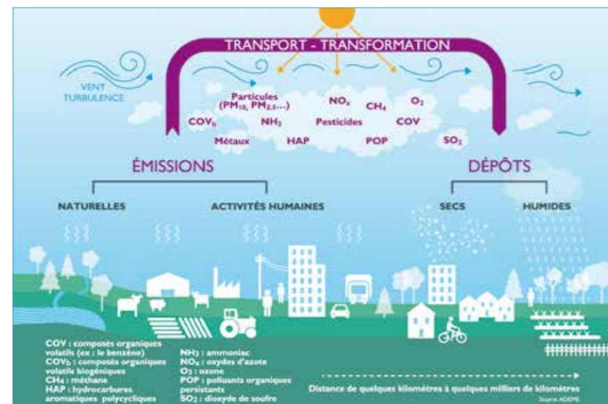
Emissions, transport, transformation, dépôts : la pollution de l'air est le résultat d'un ensemble de phénomènes complexes
