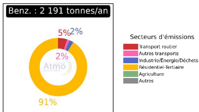
Figure 9 : Émissions de benzène (C 6 H 6 ) en 2015 dans la région Hauts-de-France.
