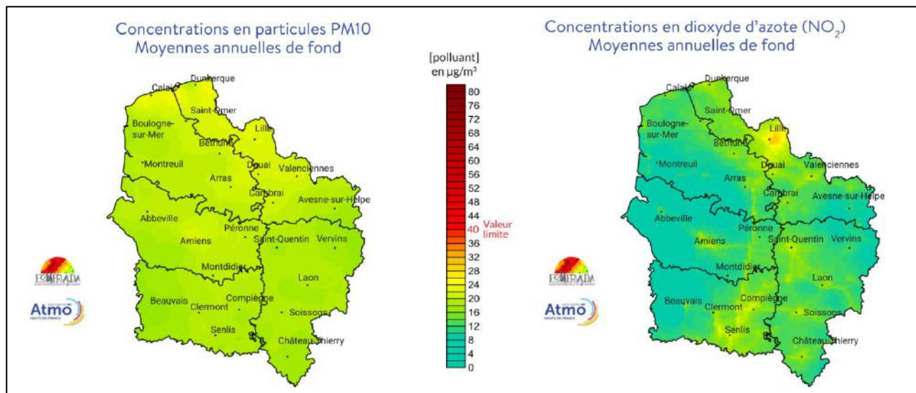
Figure 14 : Moyennes annuelles 2018 en PM 10 (à gauche) et NO 2 (à droite) modélisées pour la région Hauts-de-France.
