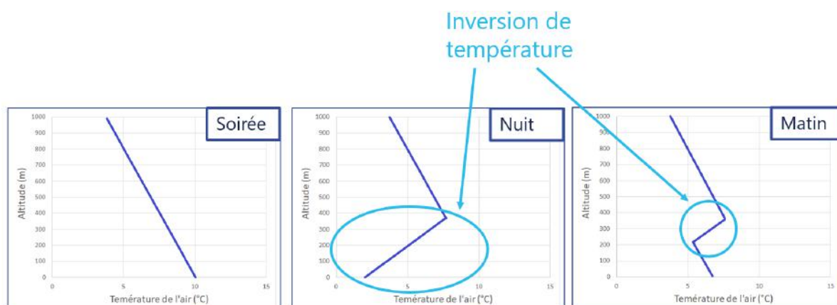
Figure 17 : Représentation schématisée de la formation d'une inversion de température par refroidissement de l'air par le sol. Sur chaque graphique est représentée la température de l'air sur l'axe des abscisses et l'altitude sur l'axe des ordonnées.
