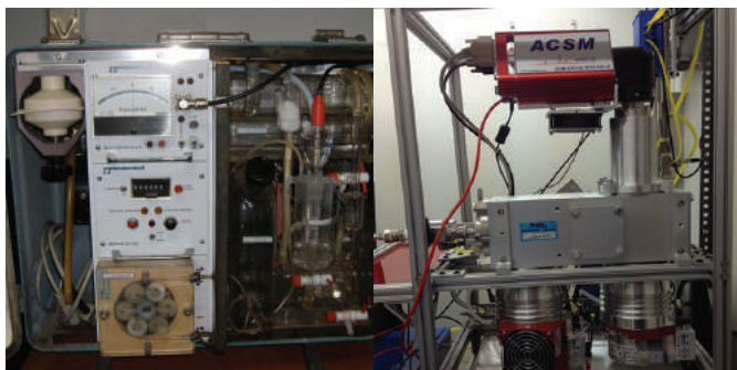
A gauche un SF2 qui mesurait l'acidité de l'air et à droite l'ACSM qui mesure la composition des particules
