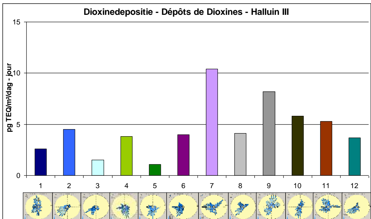
Illustration 57: Dépôt de dioxines et direction du vent au cours de la période d'échantillonnage pour les 12 campagnes de mesure, site de mesure Halluin III
