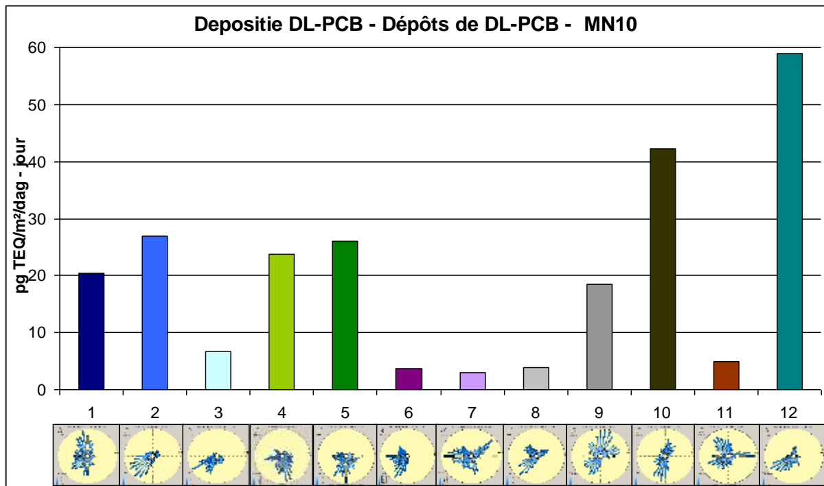
Illustration 44: Dépôt de PCB-DL et direction du vent au cours de la période d'échantillonnage pour les 12 campagnes de mesure, site de mesure MN10 (Menin)
