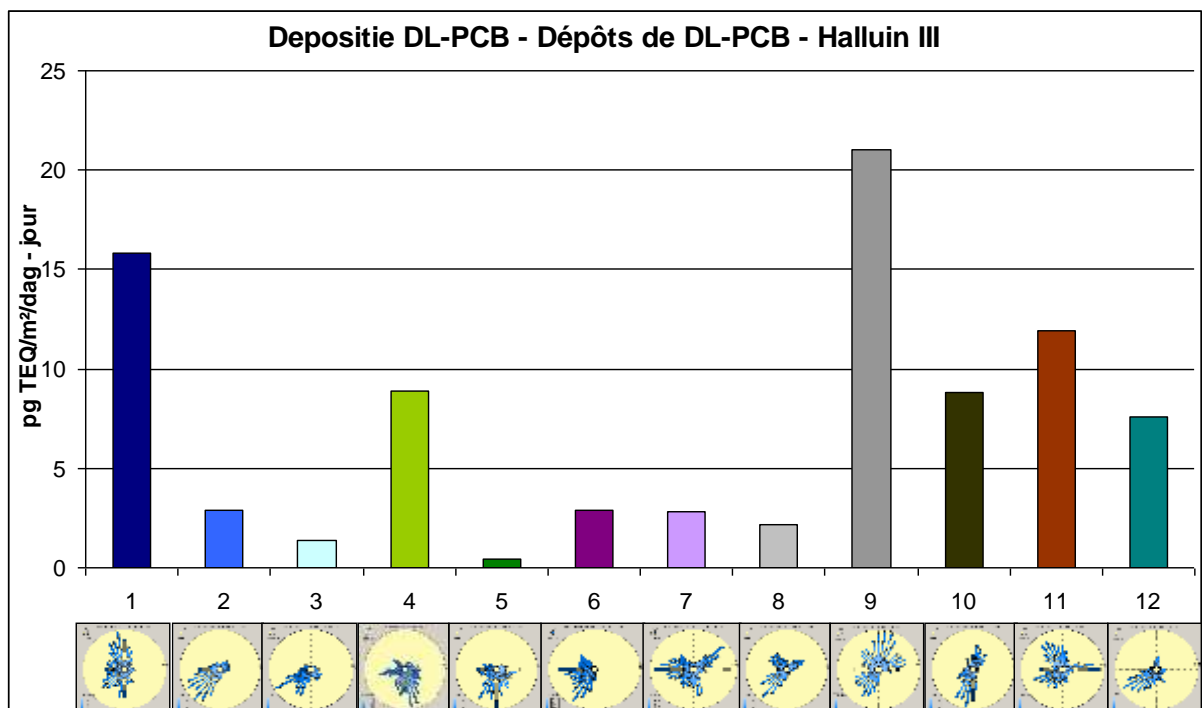
Illustration 58: Dépôt de PCB-DL et direction du vent au cours de la période d'échantillonnage pour les 12 campagnes de mesure, site de mesure Halluin III
