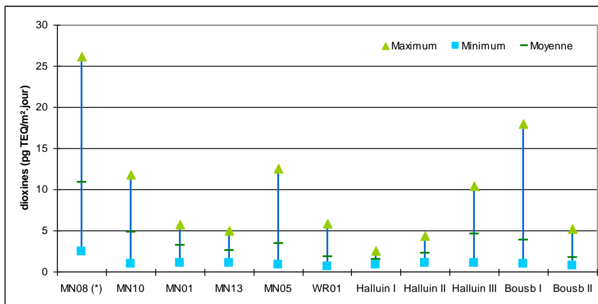
Illustration 27: Dépôt de dioxines par site de mesure : moyenne, minimum et maximum observés pendant les campagnes de mesure mensuelles
