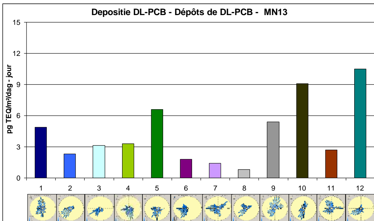
Illustration 48: Dépôt de PCB-DL et direction du vent au cours de la période d'échantillonnage pour les 12 campagnes de mesure, site de mesure MN13 (Menin)
