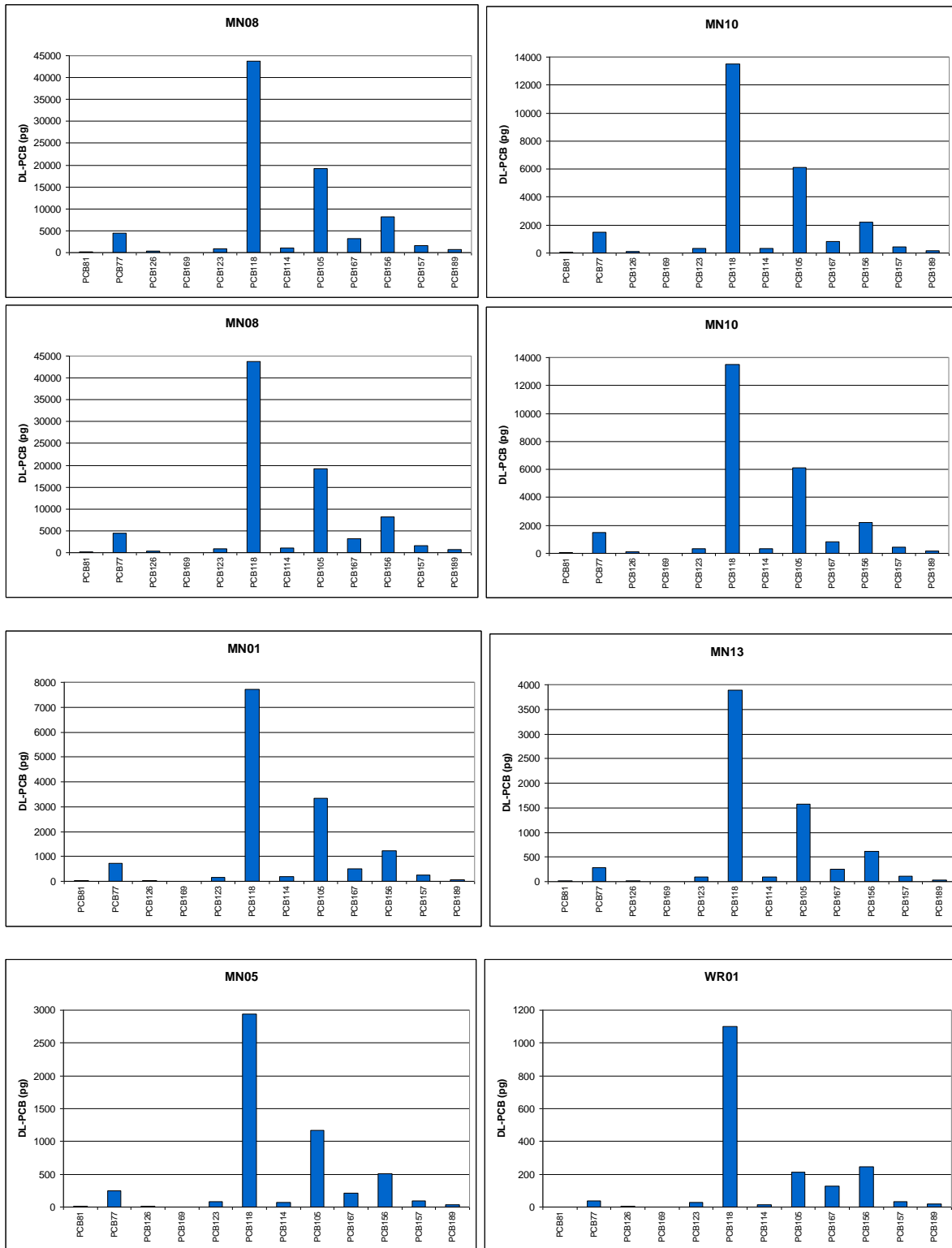
Illustration 36: Profils moyens de 12 congénères de PCB-DL, pour les 12 campagnes de mesure (période juillet 2011 – juillet 2012), sites de mesure de Menin (MN) et Wervik (WR) NB : les échelles peuvent être différentes d'un graphique à un autre.
