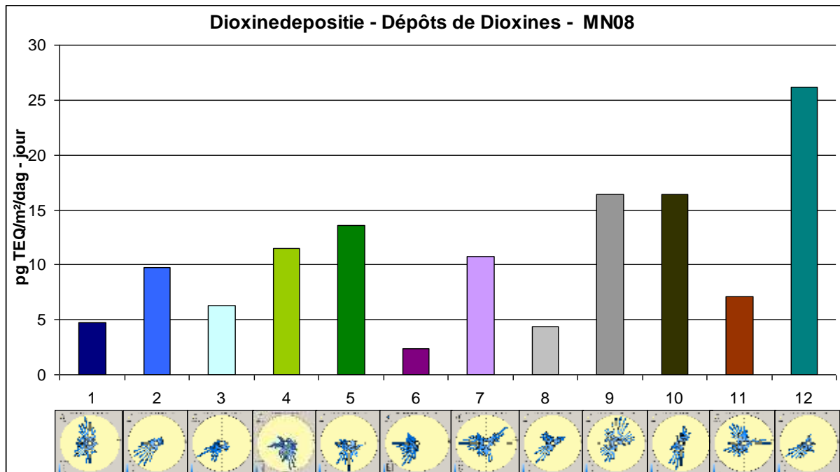
Illustration 41: Dépôt de dioxines et direction du vent au cours de la période d'échantillonnage pour les 12 campagnes de mesure, site de mesure MN08 (Menin)
