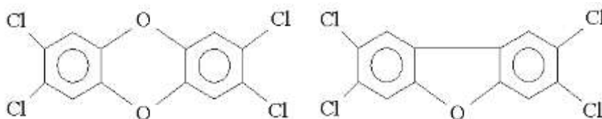
Illustration 1: Formule chimique des molécules PCDD et PCDF
