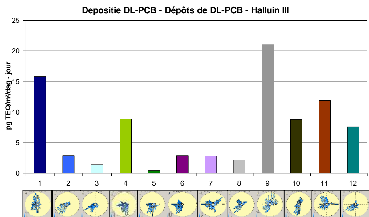
Illustration 32: Dépôt de PCB-DL et roses des vents associées pour les 12 campagnes de mesure, site de mesure Halluin III
