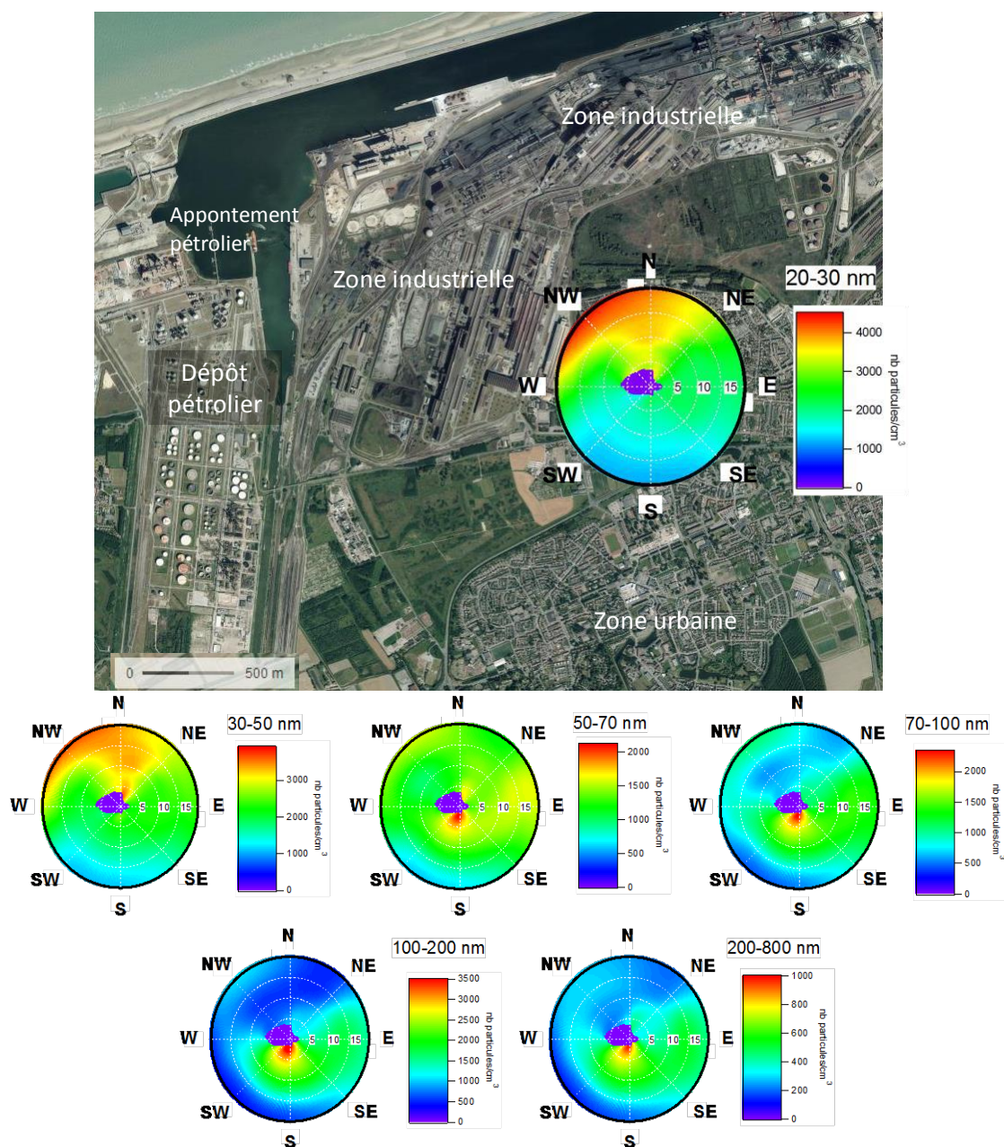
Figure 36 Roses de pollution pour 6 classes de tailles de particules (phase 2)
