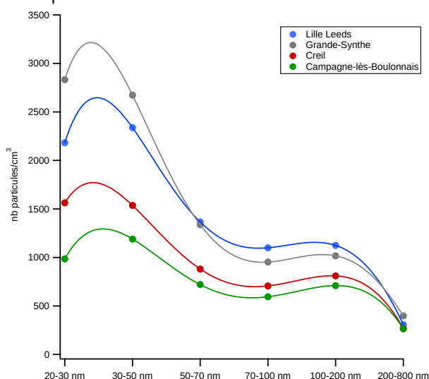
Figure 1 Distribution des tailles de PUF pour les 4 sites étudiés
