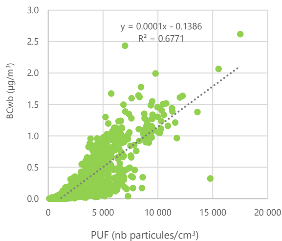
PUF et BC wb : Campagne-lès-Boulonnais (phase 2)
