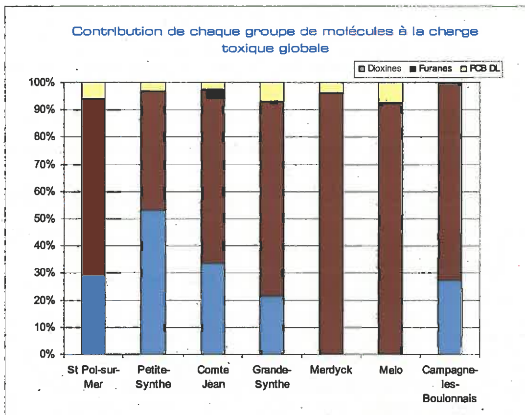
Figure 26 : Contribution à la charge toxique globale exprimée en pg I-TEQ OMS /m 2 /j
