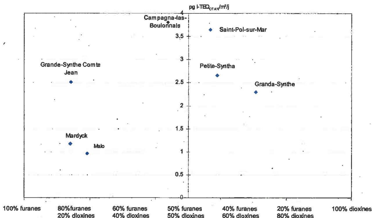
Figure 18 : Répartition des équivalents toxiques en fonction du profil Dioxines/Furanes dans les retombées
