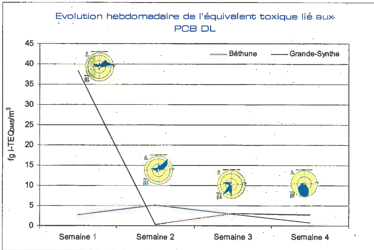
Figure 34 : Concentrations de PCB DL en équivalent toxique exprimée en fg I-TEQOMS/m 3
