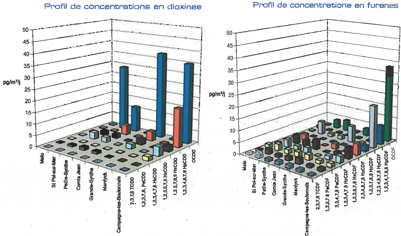
Figure 17 : Concentrations en dioxines et furanes dans les retombées ( \text{pg}/\text{m}^2/\text{j} )
