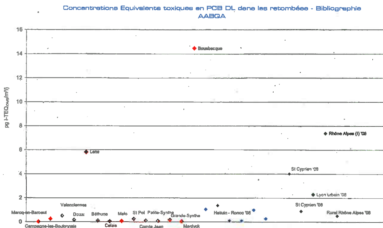
Figure 23 : Bibliographie disponible pour les équivalents toxiques en PCB DL dans les retombées (pg/m 2 /j)
