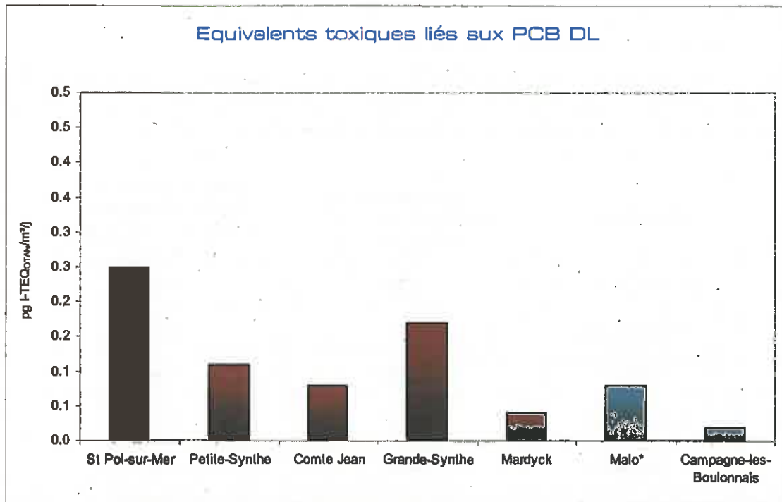
Figure 21 : Concentrations en équivalents toxiques en PCB DL dans les retombées (I-TEQOMS pg/m²/j)
