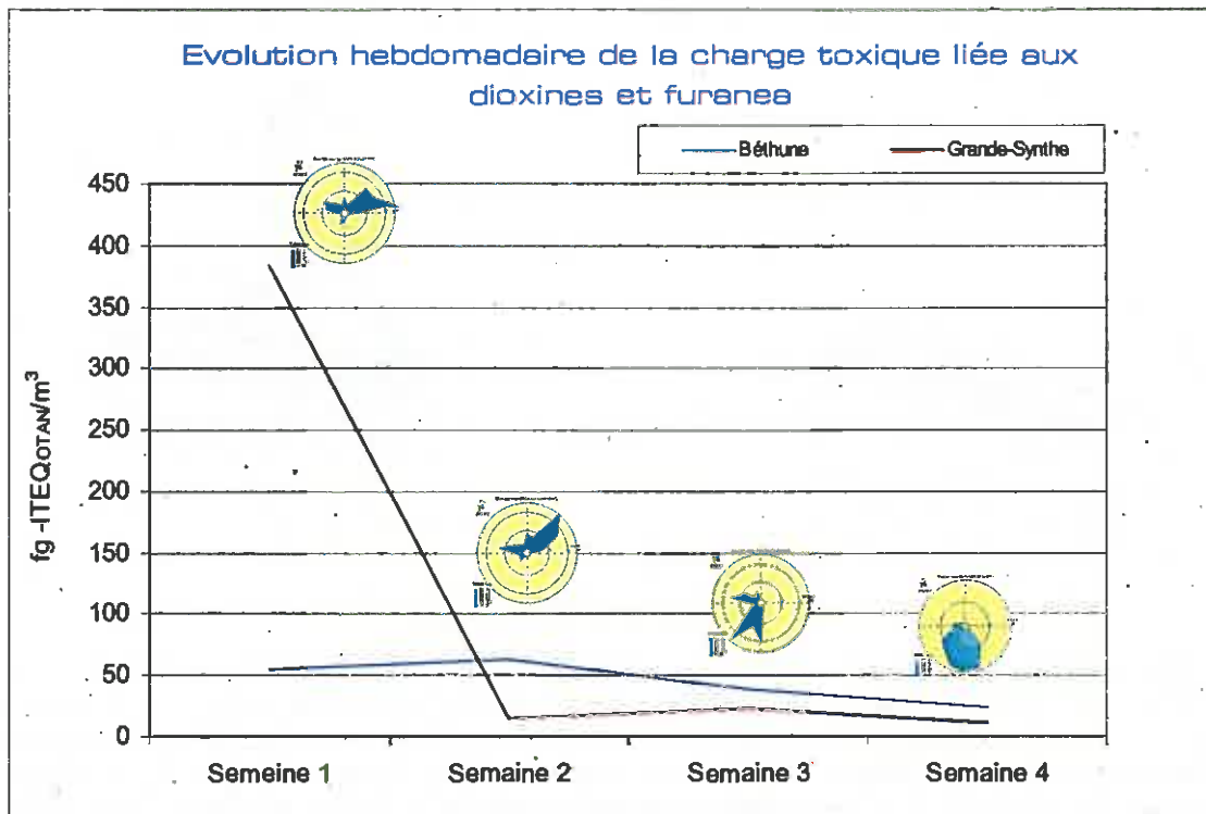
Figure 28 : Concentration hebdomadaire en équivalent toxique exprimée en fg I-TEQOTAN/m 3
