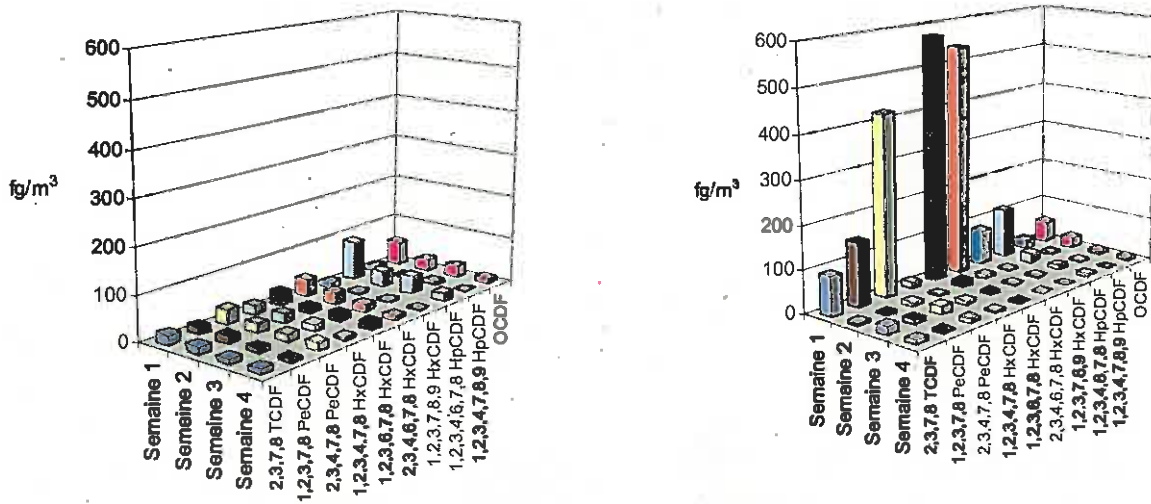
Figures 30 : Profils de concentrations en furanes
