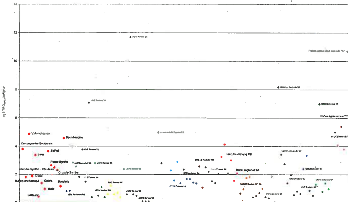
Figure 19 : Comparaison à la bibliographie disponible auprès des AASQA
