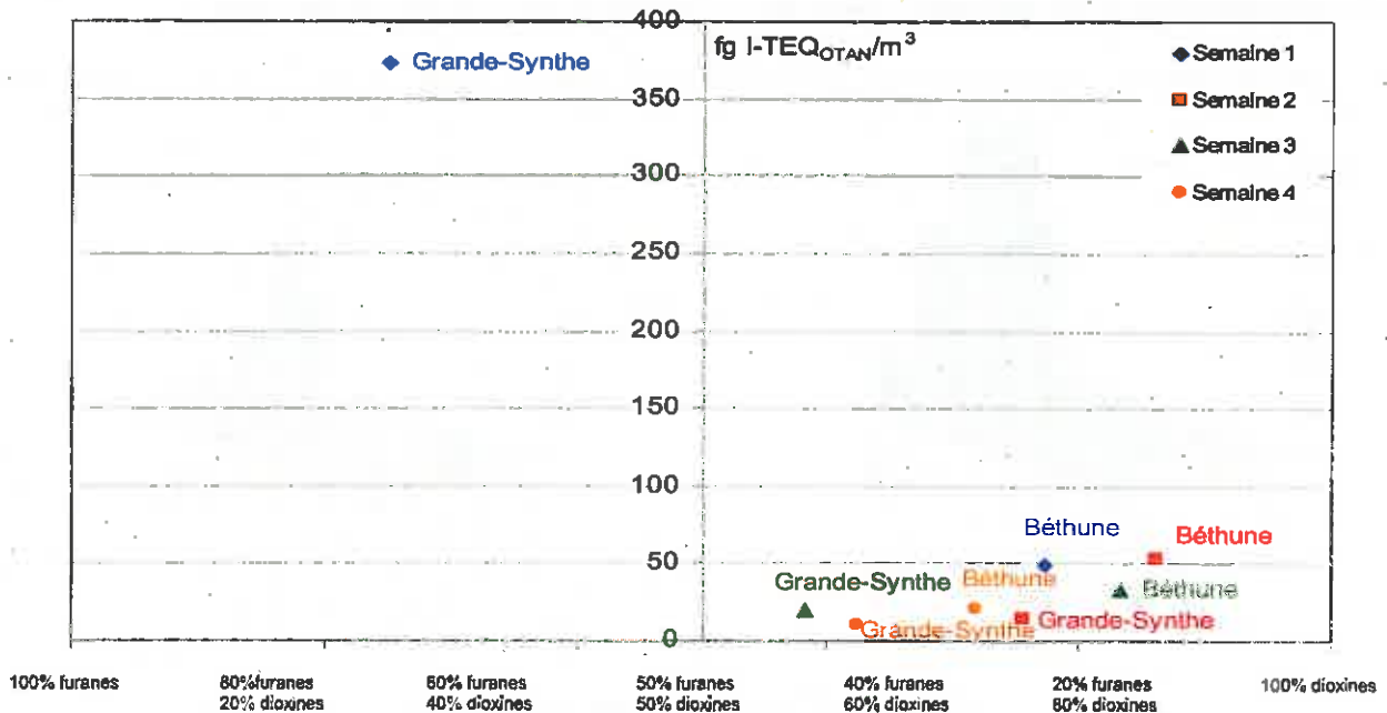
Figure 31 : R partition de l’ quivalent toxique en fonction du profil Dioxines /Furanes en air ambiant
