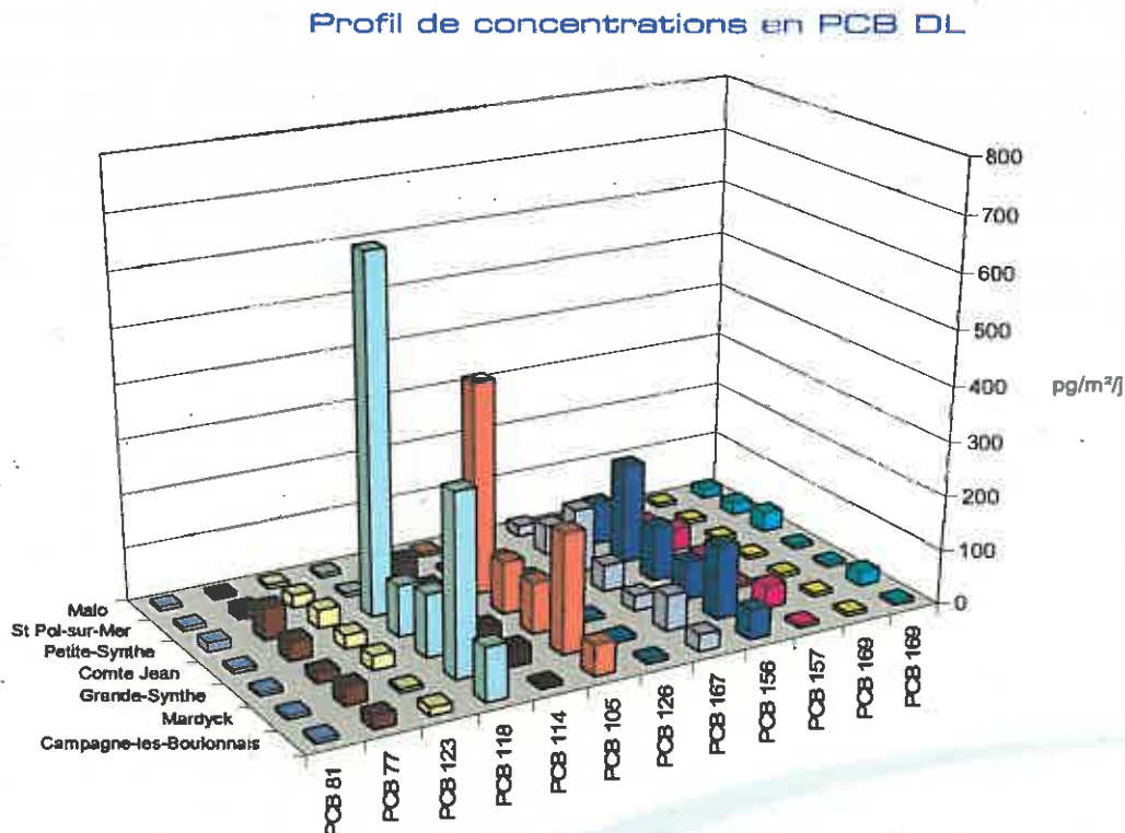
Figures 22 : Concentrations en PCB DL dans les retombées (pg/m²/j)
