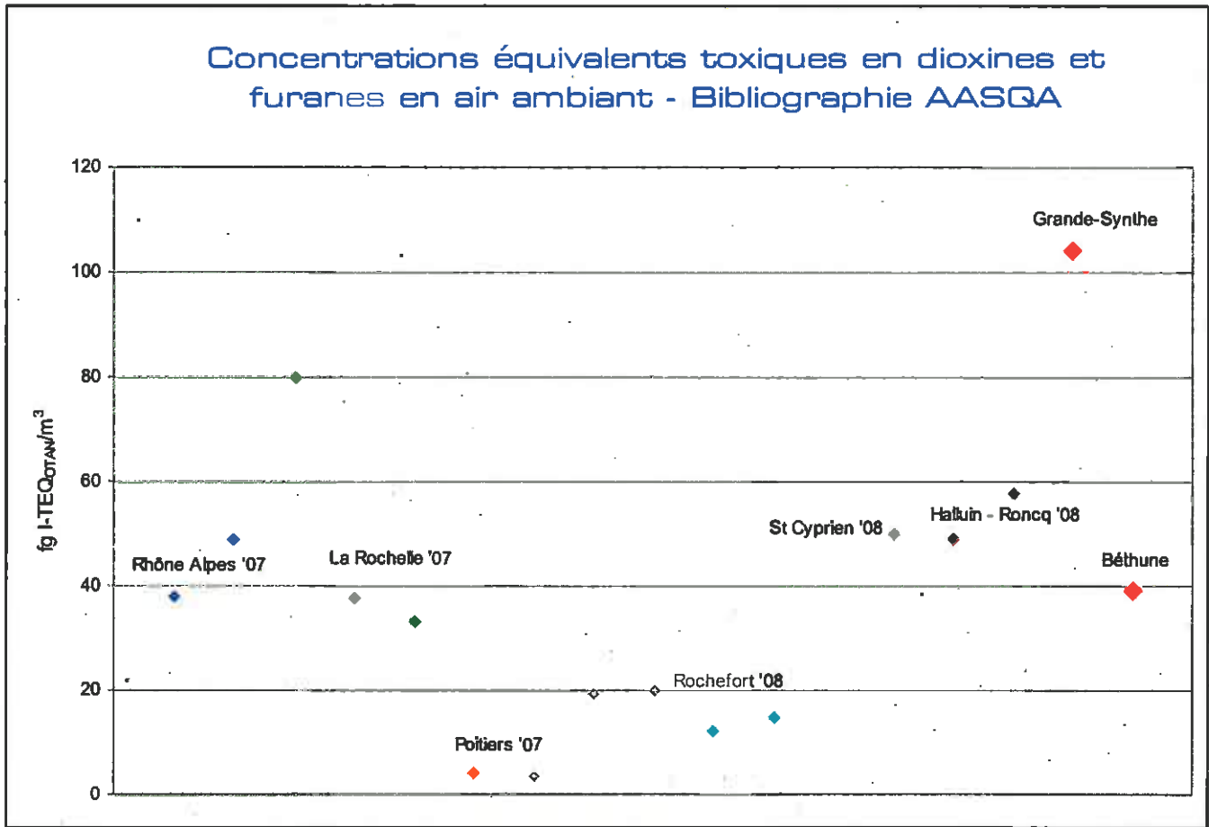
Figure 32 : Bibliographie nationale des concentrations dioxines furanes en air ambiant
