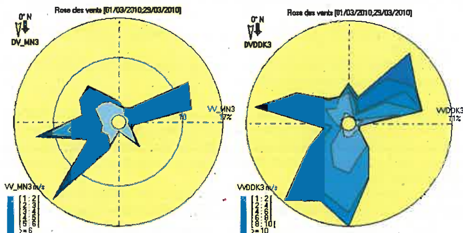
Figure 13 : Roses des vents (Tourcoing à gauche, Dunkerque à droite)
