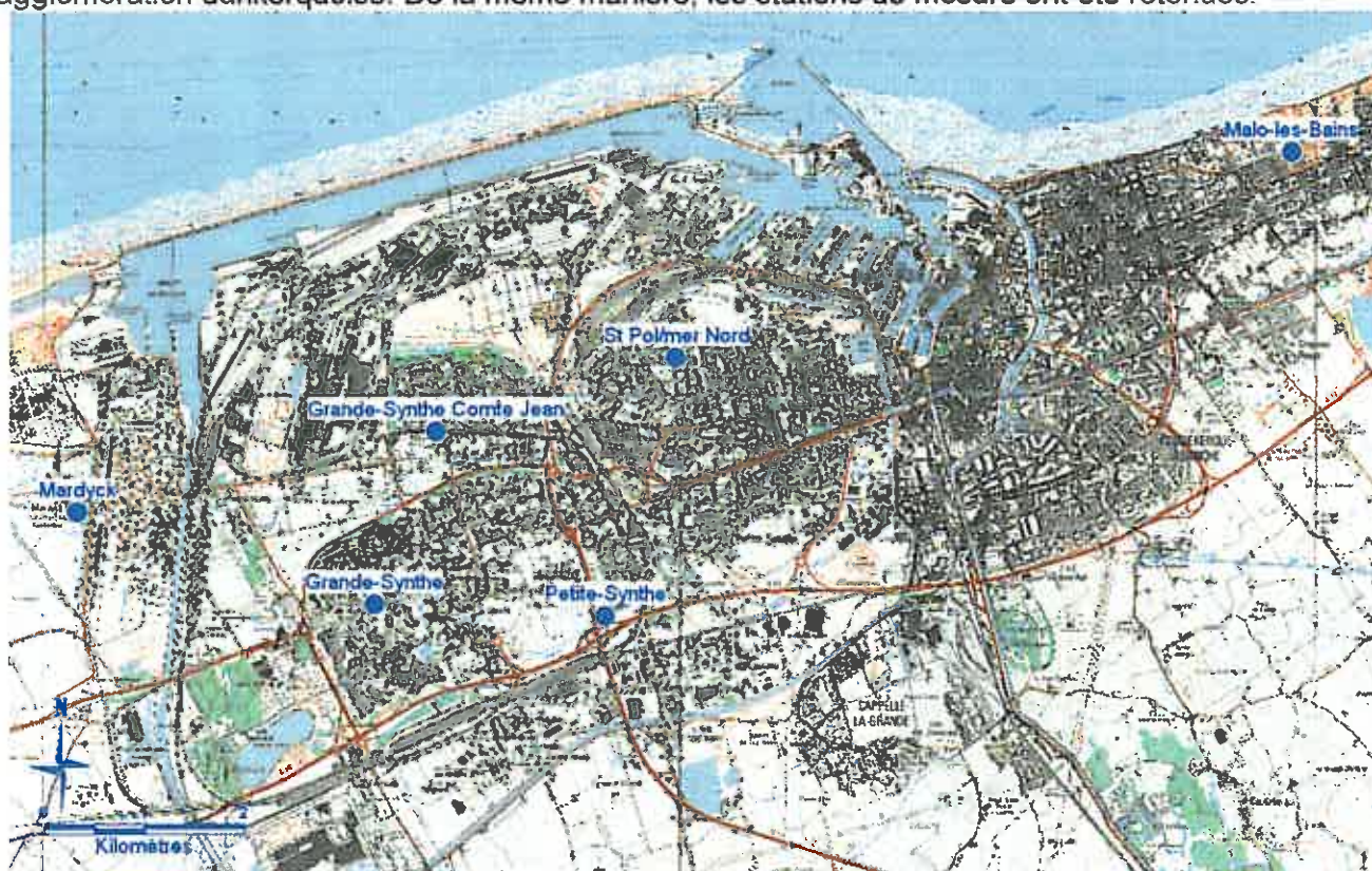
Figure 10 : Carte de localisation des sites de prélèvement sur le dunkerquois
