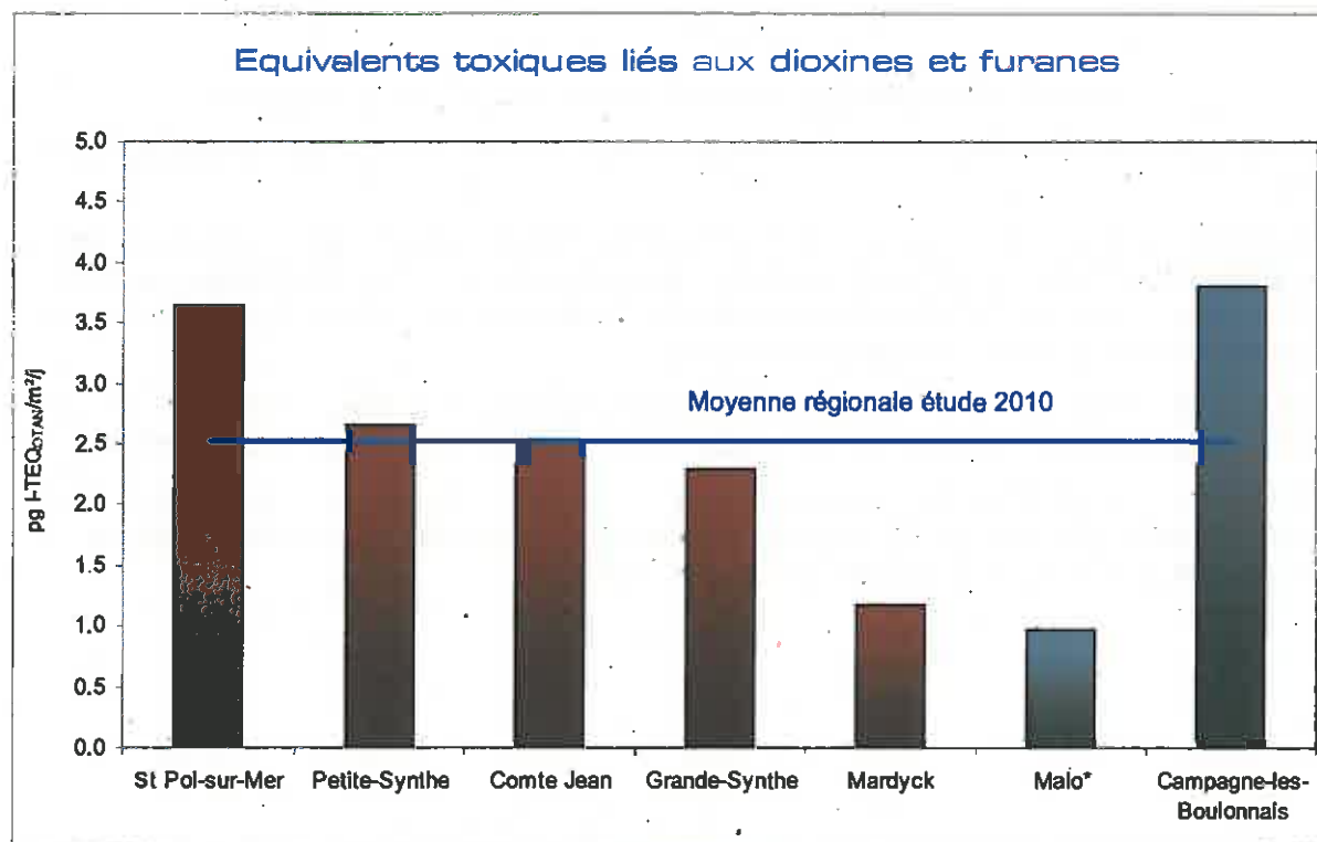
Figure 16 : Equivalents toxiques en dioxines furanes dans les retombées (I-TEQ OTAN pg/m 2 /j) sur l'agglomération dunkerquoise
