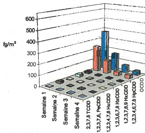
Figures 29 : Profils de concentrations en dioxines
