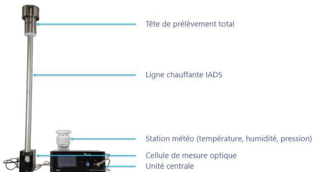
Analyseur FIDAS 200. Source : ADDAIR 15
