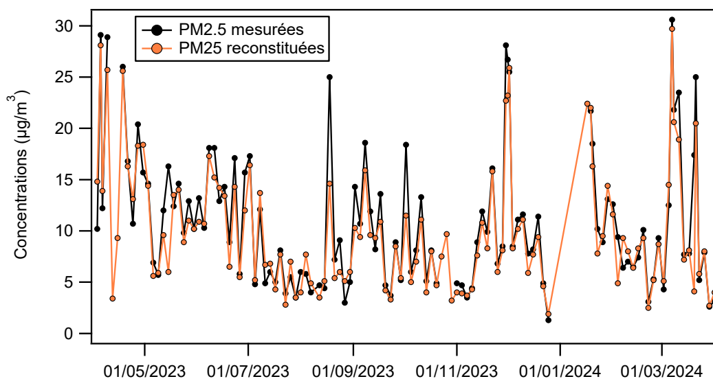
Séries temporelles des PM2.5 mesurées (noir) et reconstituées (orange) par le modèle PMF
