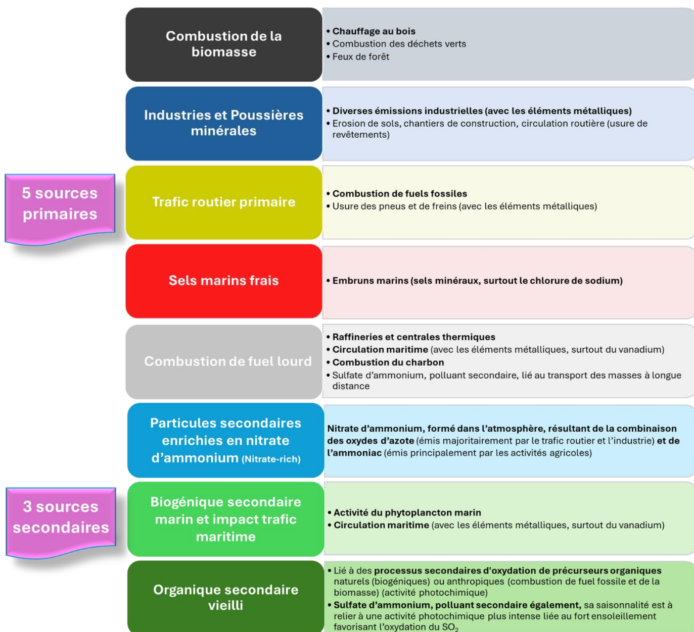
Figure 1 : Sources principales influencent les concentrations de PM2.5.
