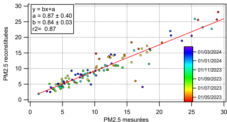
Corrélation entre les PM2.5 mesurées et les PM2.5 reconstituées par le modèle PMF
