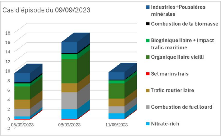
Figure 38 : Séries temporelles des différents facteurs à Lille, zoom sur la période étudiée.
