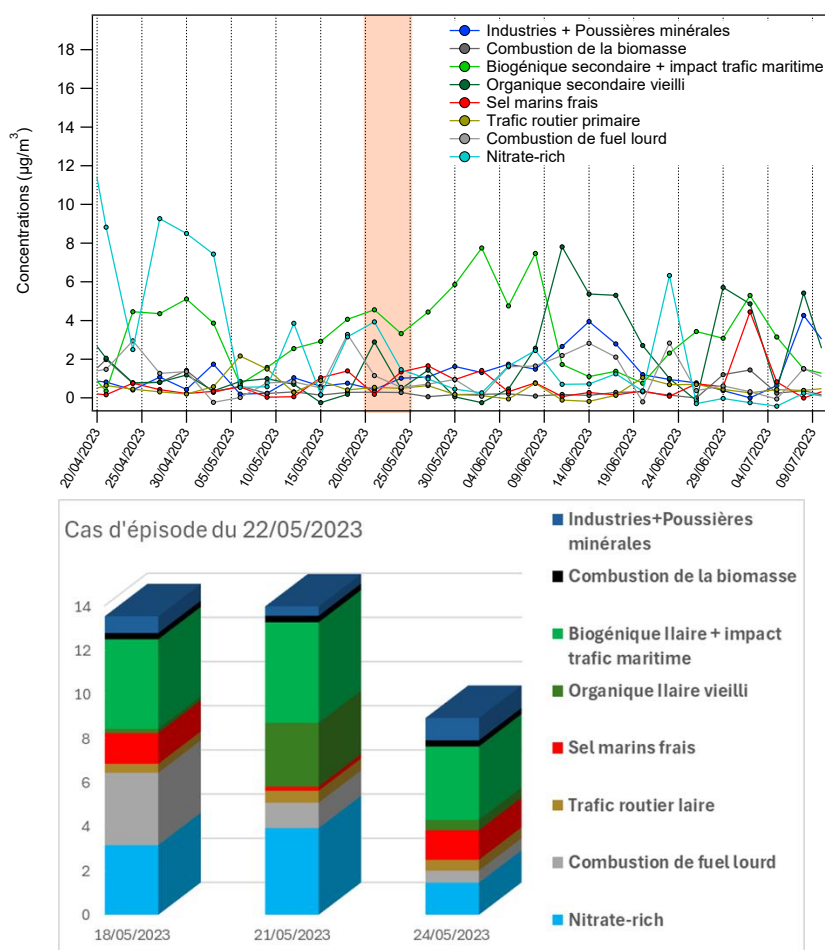
Figure 35 : Séries temporelles des différents facteurs à Lille, zoom sur la période étudiée
