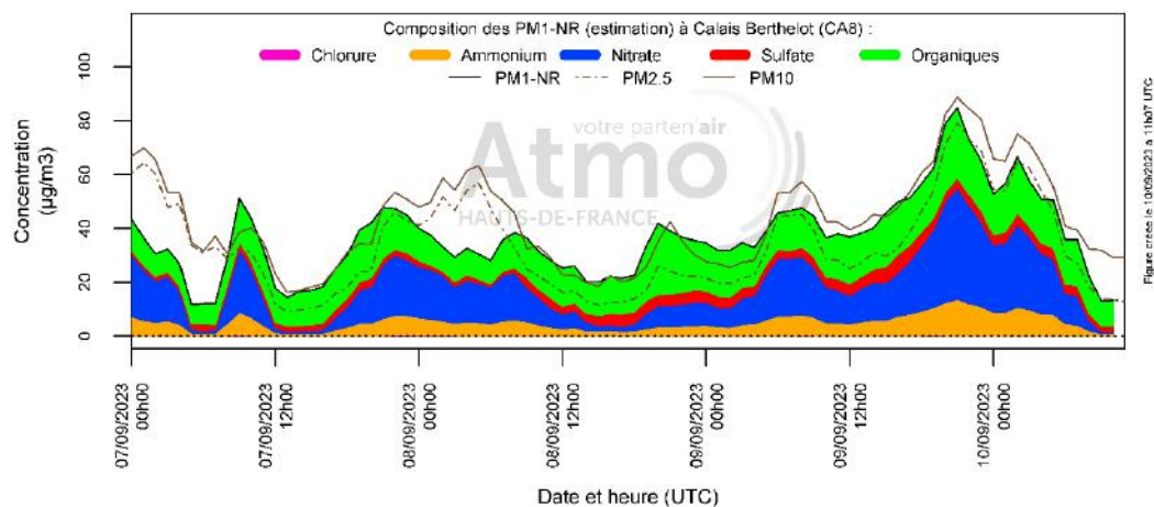
Figure 36 : données ACSM à Calais, consultées le 10/09/2023
