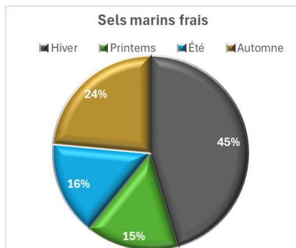
Figure 17 : Variation saisonnière de la source « Sels marins frais »
