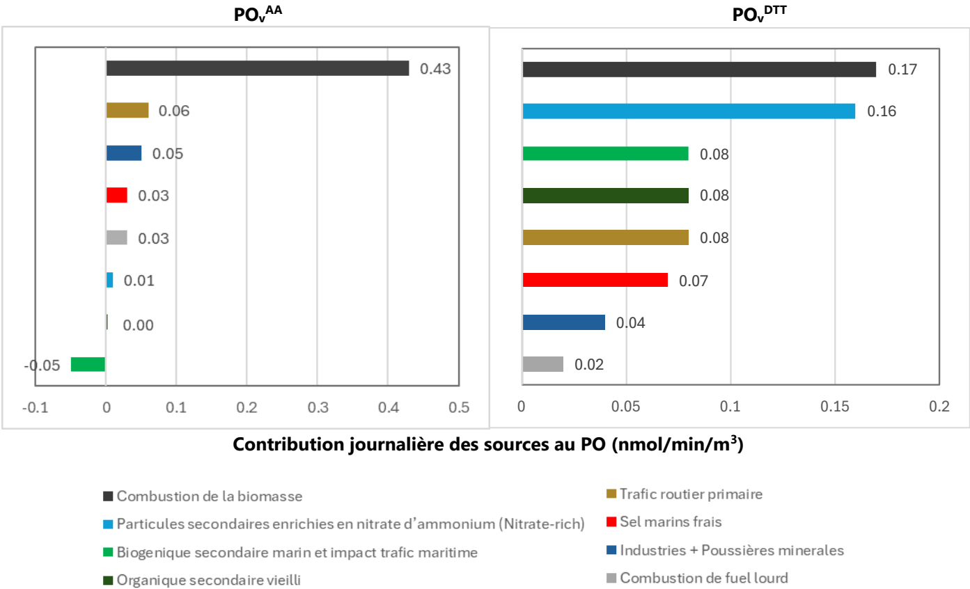
Figure 32 : Contribution moyenne et variabilité (95% d'intervalle de confiance) sur l'année des différentes sources d'émission des PM aux PO^{AA} et PO^{DTT} volumique à Lille.
